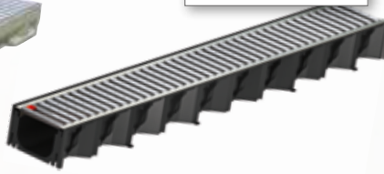
Clase A15 Conjunto de canal y tapa.
